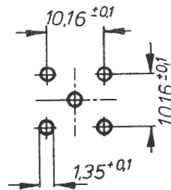
Montagedurchbrüche
