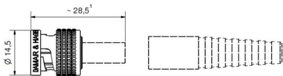
Kabelstecker mit Knickschutztüle
