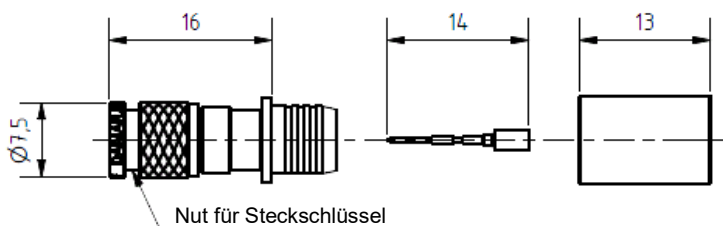
Abb.2: Kabelstecker-Ø 6 - 7 mm
