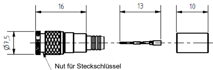
Abb.1: Kabelstecker-Ø 3 - 5
