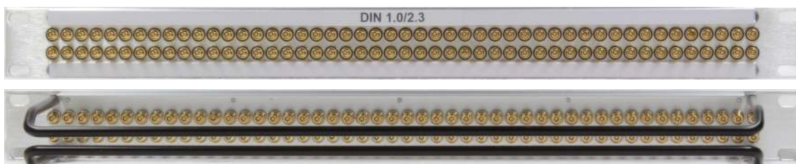
Abb. 3: DIN 1,0/2,3 Steckfeld
