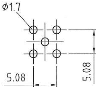
Leiterplattenlochbild
