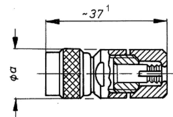
Kabelstecker mit zusätzl. Kabelzugentlastung 1 Gesamtlänge
